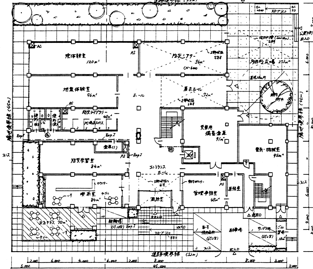
1階平面図 未配置図 1/200
