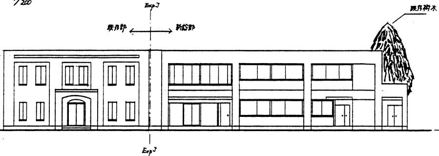
立面図 1/200
