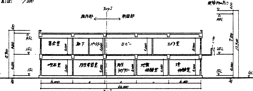
断面図 1/200
