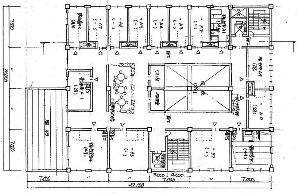
(3) 3階平面図 (S:1/200)
