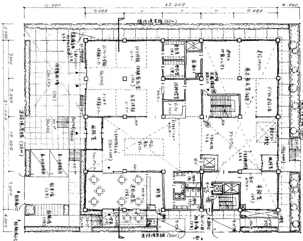
1階平面図 床配置図 S = 1/200
