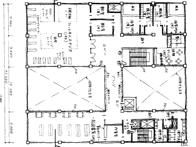
3階平面図 S = 1/200
