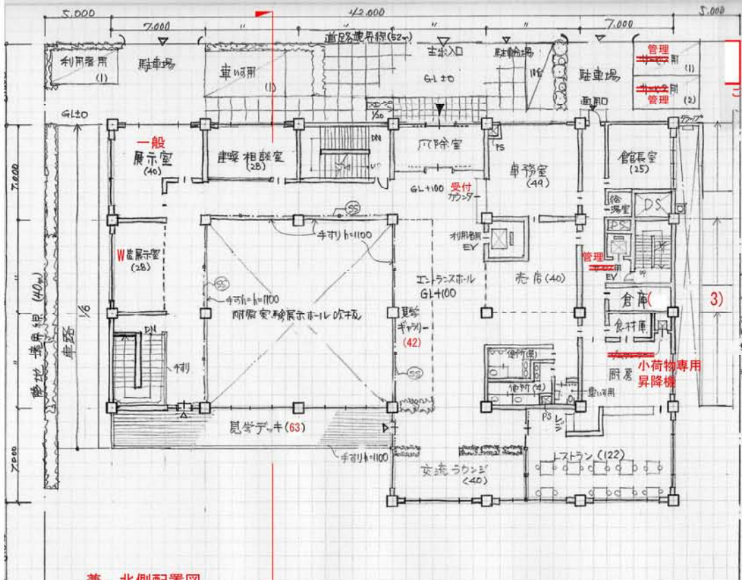
兼 北側配置図
