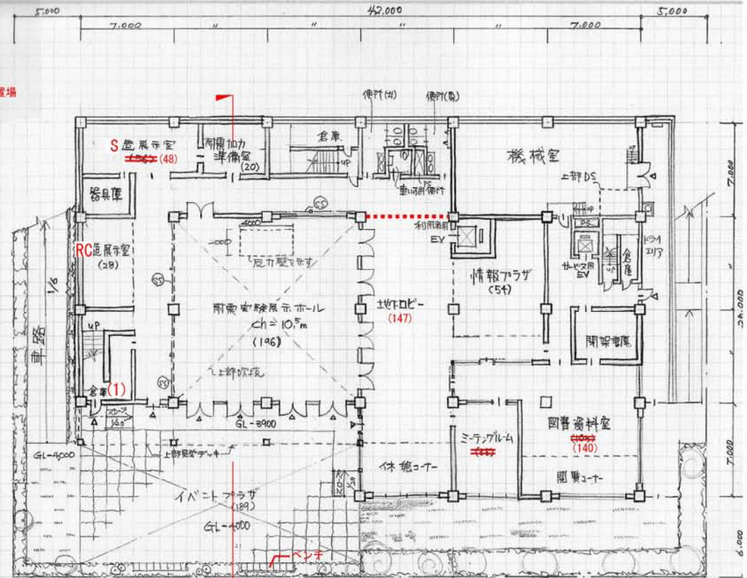
地下1階平面図 1/200
